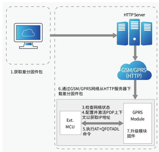
▲ 图 1: 通过 DFOTA 从 HTTP 服务器升级固件
